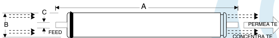
ElementDetails**
